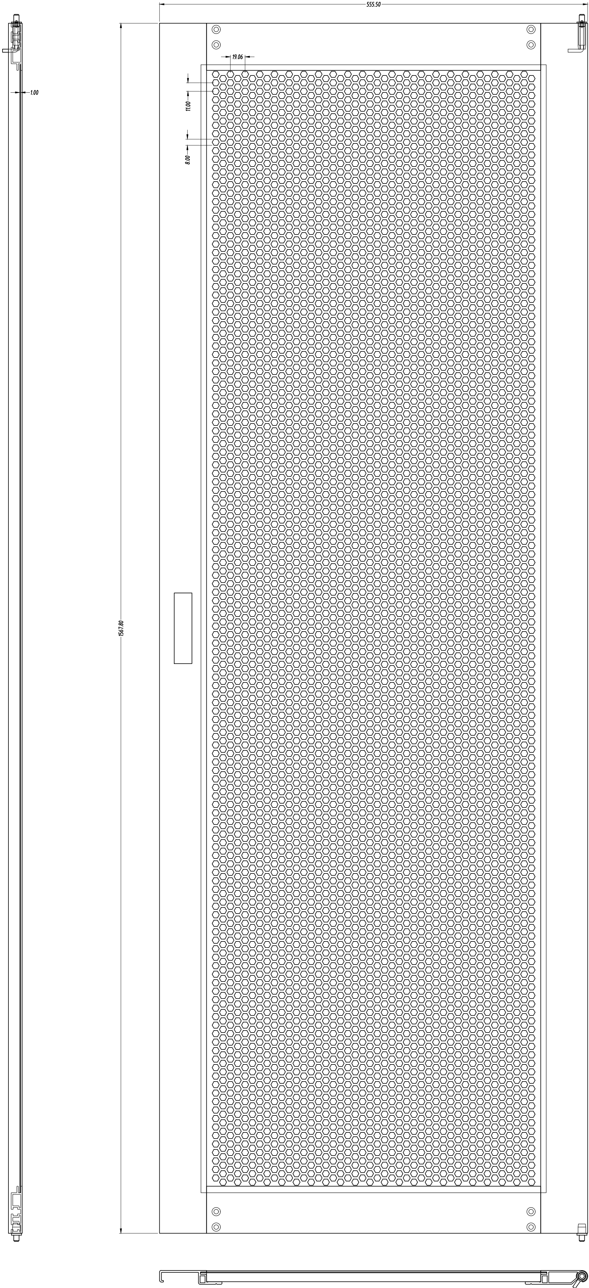
35U机柜后门尺寸：1567.8*555.5*18mm
