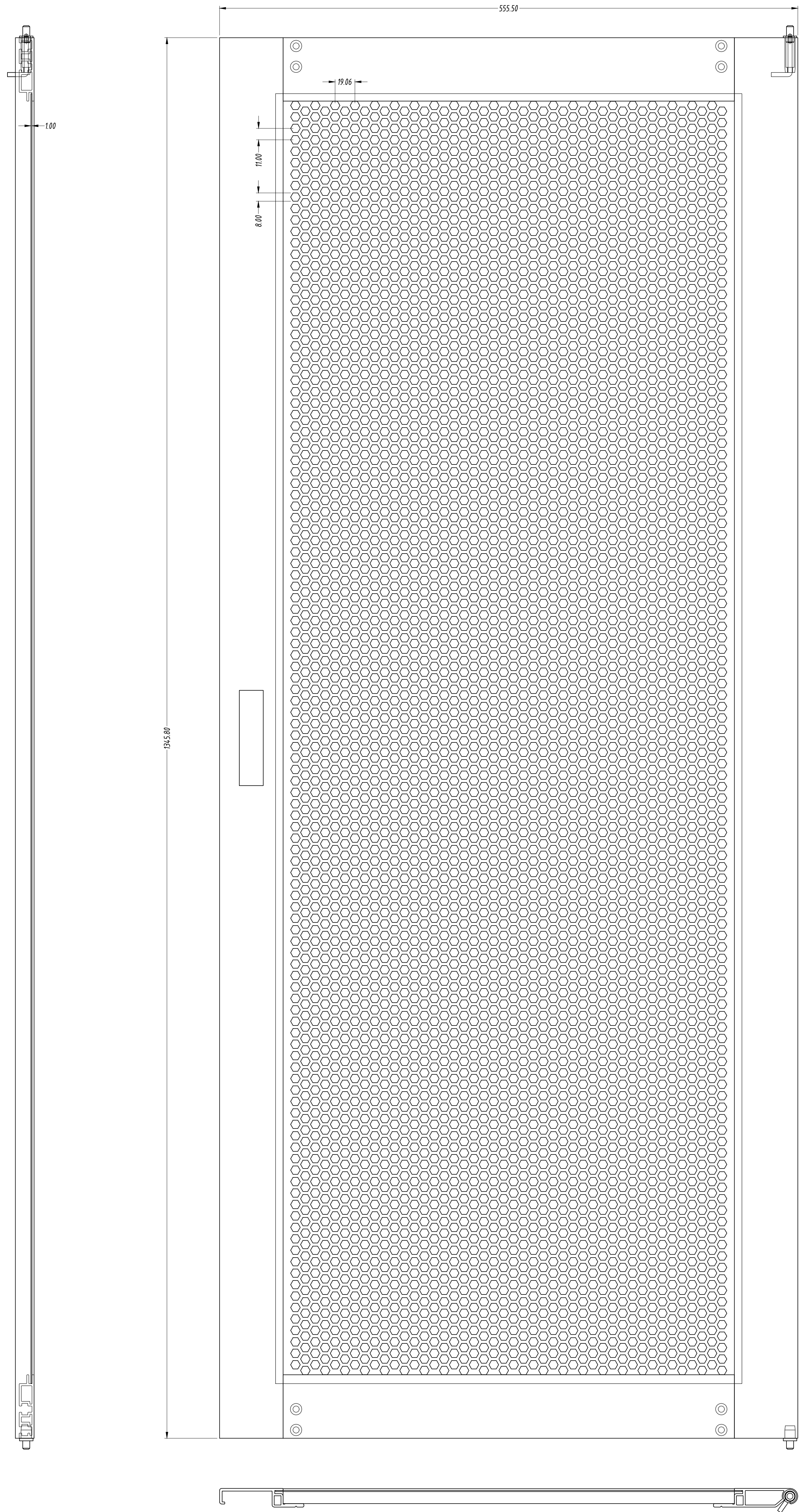
30U机柜后门尺寸：1345.8*555.5*18mm
