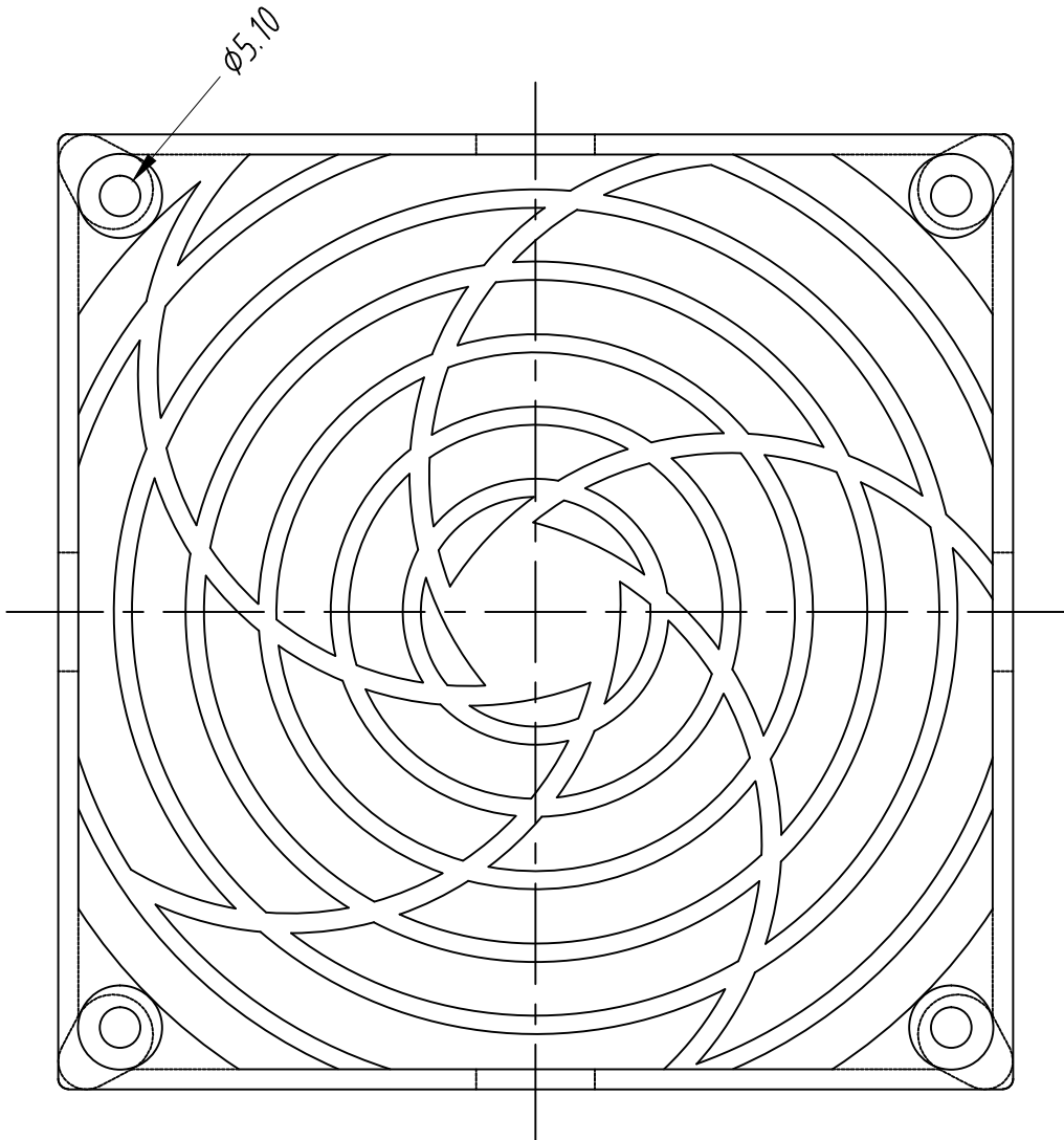
十二公分三合一保護網下蓋
