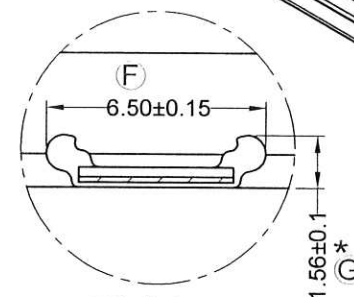
局部放大圖 B 5:1
