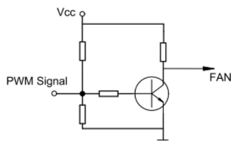
PWM control circuit PWM控制接口电路
