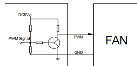
PWM control circuit PWM控制接口电路
