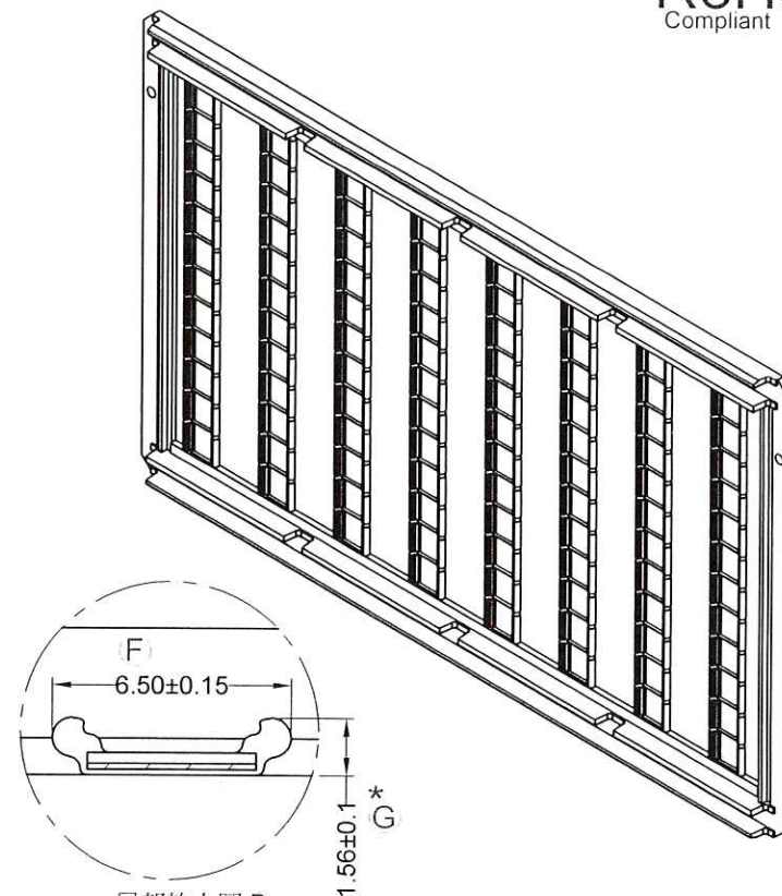
局部放大圖 B 5:1
