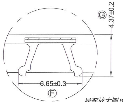
局部放大圖 B
