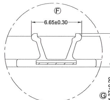
局部放大圖 B 5:1
