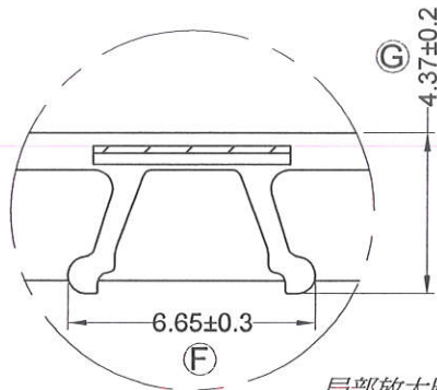
局部放大圖B
