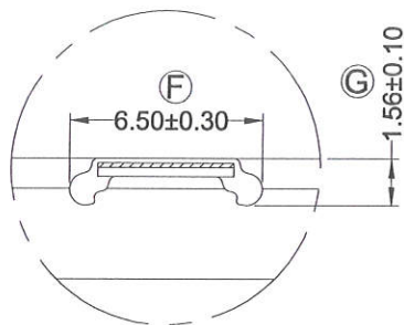
局部放大圖 B
